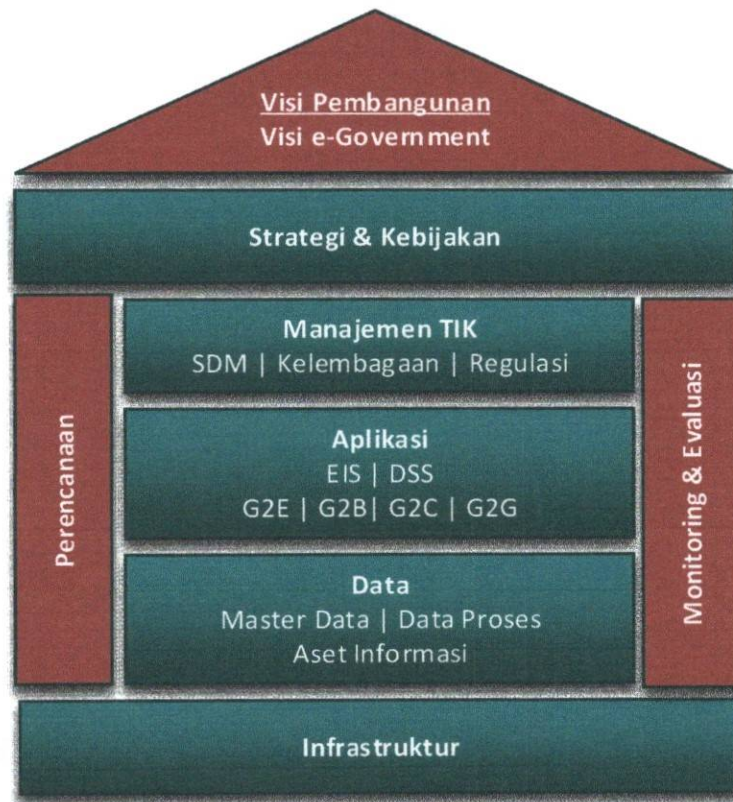
Gambar 1. Arsitektur e-Government
